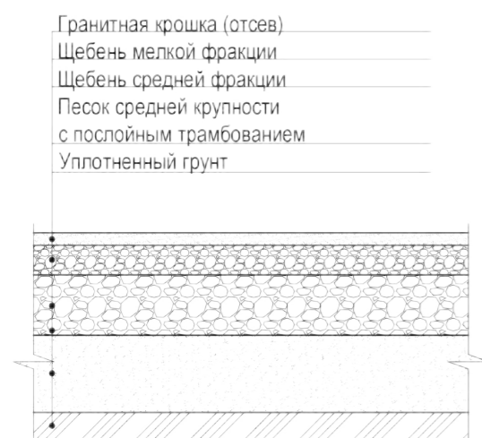
3.6 схема устройства основания под набивное покрытие
